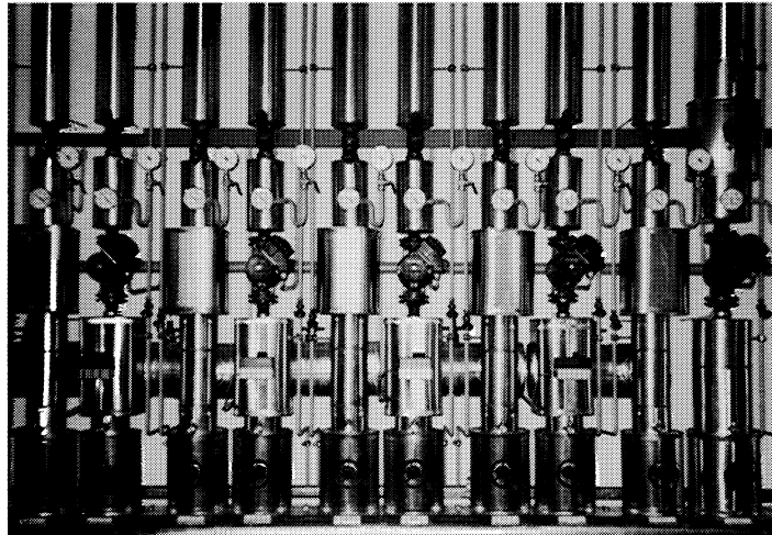
Die neue Fernwärmeheizung in Carl-Jacob-Burkhardt-Gymnasium in Lübeck
